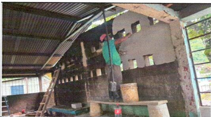
FOTO 10: Reparación y cernido de paredes
